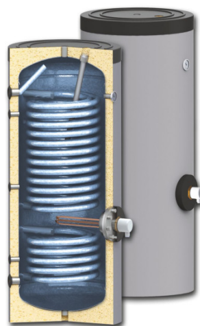
Boiler SWPN2 cu doua serpentine
