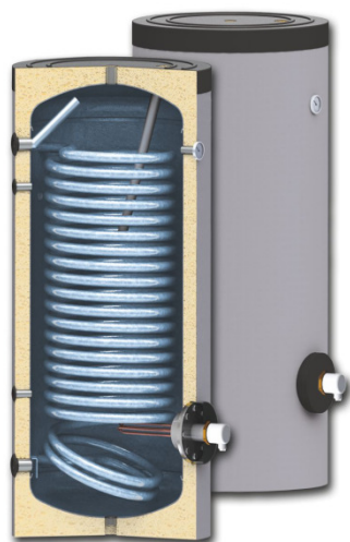
Boiler SWPN cu o serpentina
